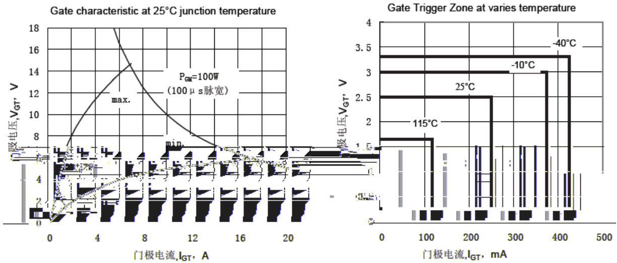
门极功率曲线
