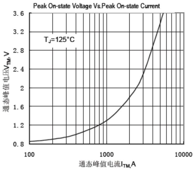
安特性曲线
