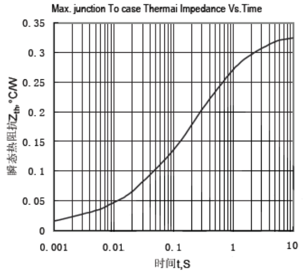
Fig.2 结至管壳瞬 热阻抗曲线
