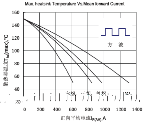
Fig.6 散热器温度与 态平均电流关系曲线
