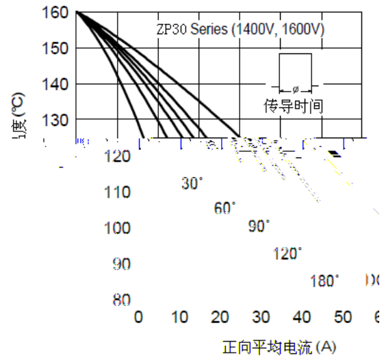
Fig. 4 - 额定电流特性
